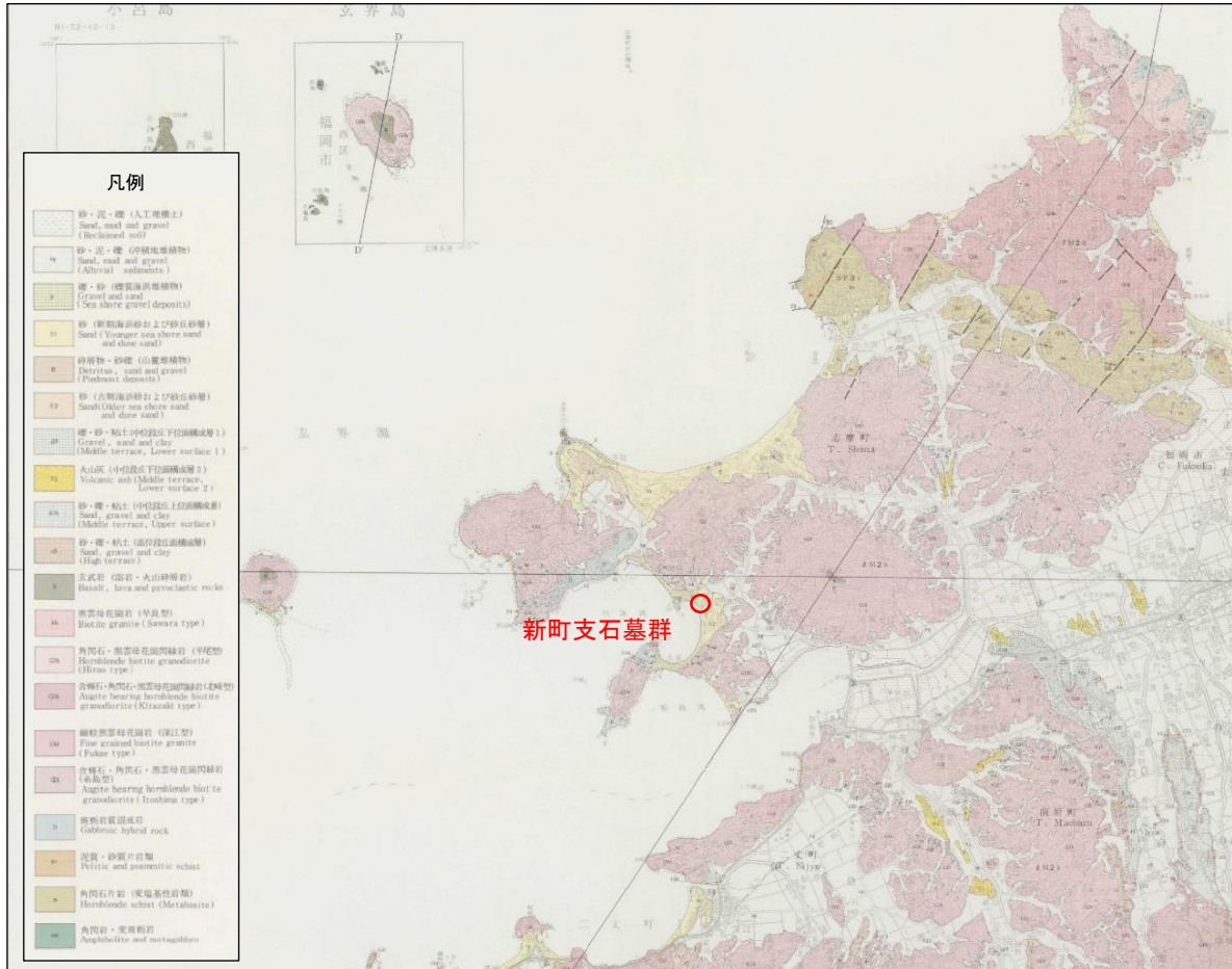
図 2-3 表層地質図
