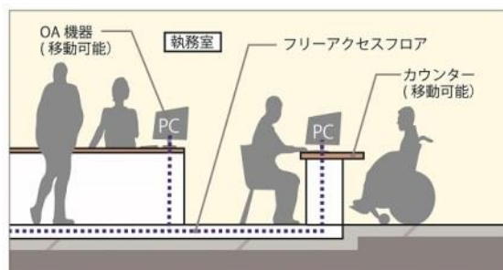
フリーアクセスフロアイメージ
